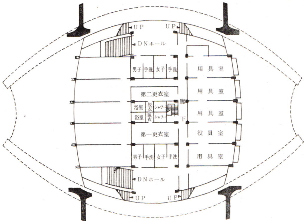
2 階 平 面 図
